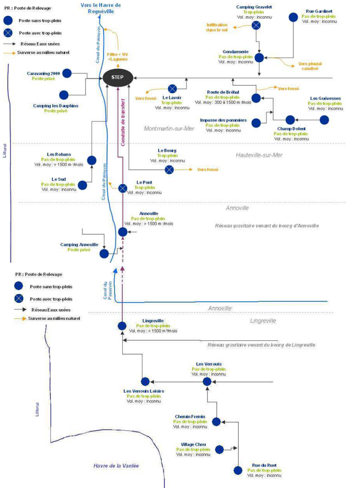
Figure 61 : Schéma conceptuel des réseaux d'assainissement sur le territoire du Syndicat Intercommunal de Traitement des Eaux Usées (SITEU) de Montmartin-sur-Mer, Hauteville-sur-Mer, Annoville et Lingreville.
