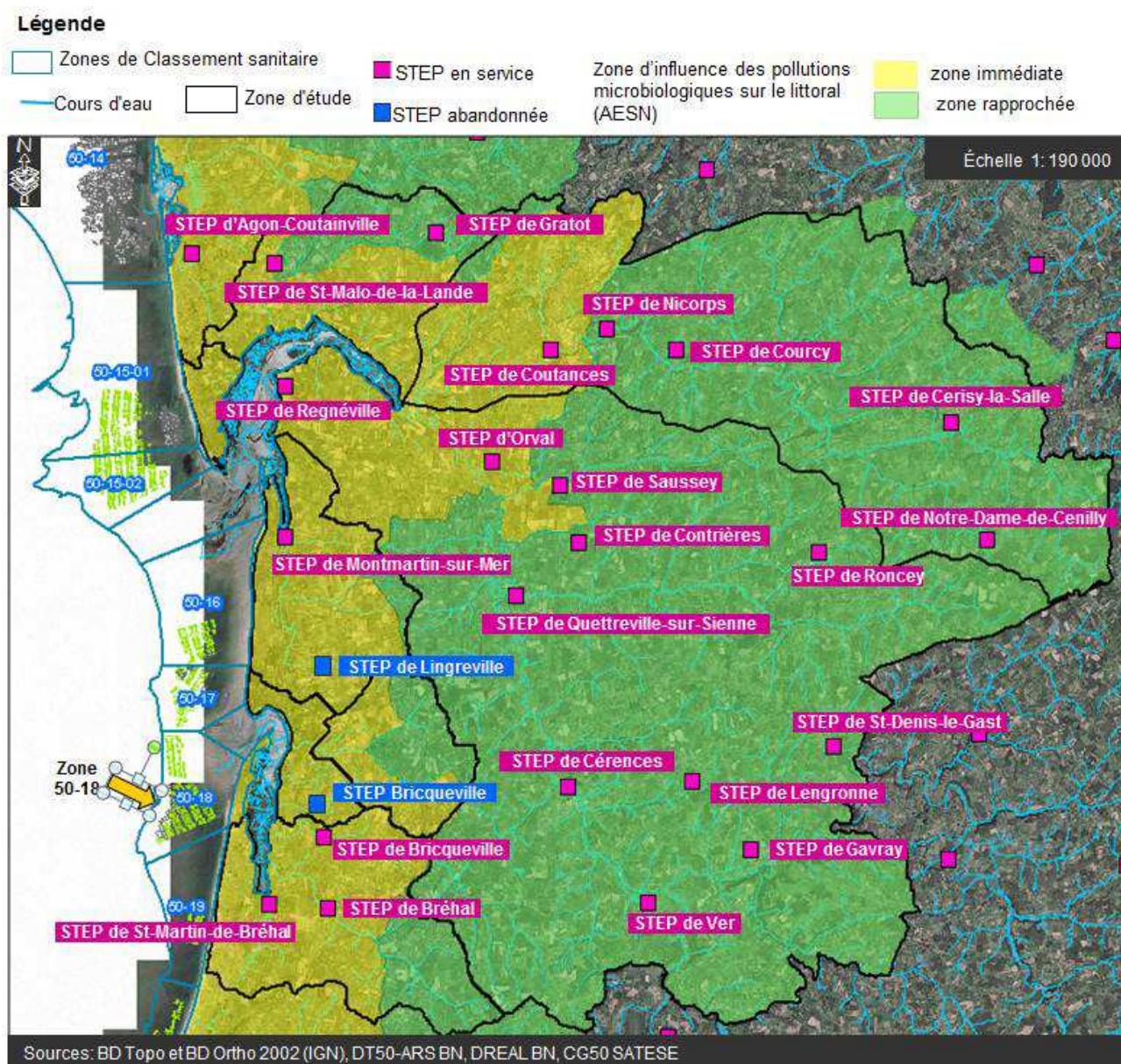
Figure 49 : Localisation des stations d'épuration sur la zone d'étude
