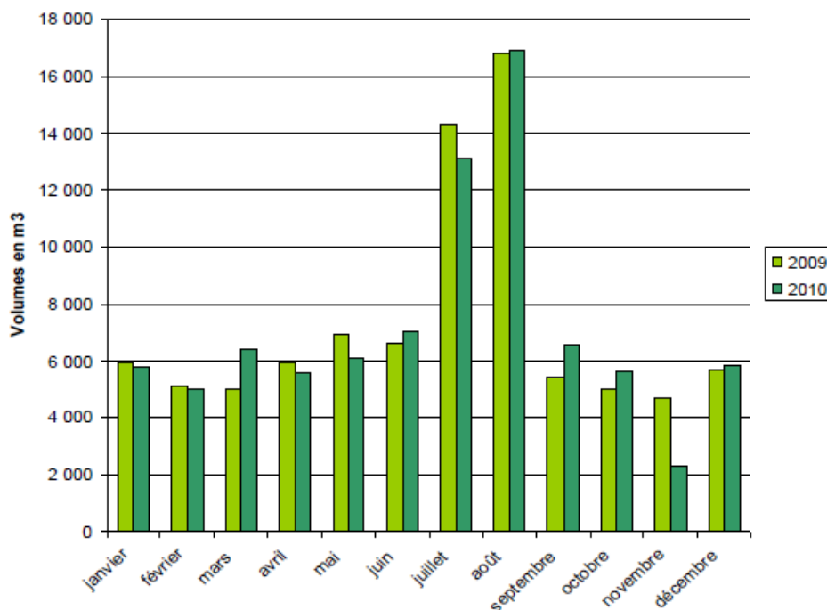
Figure 68 : Evolution des volumes d'eaux usées traitées par la station de Saint-Martin-de-Bréhal en 2009 et 2010 Graphique extrait du rapport technique STGS fourni à la commune (STGS, 2010).
