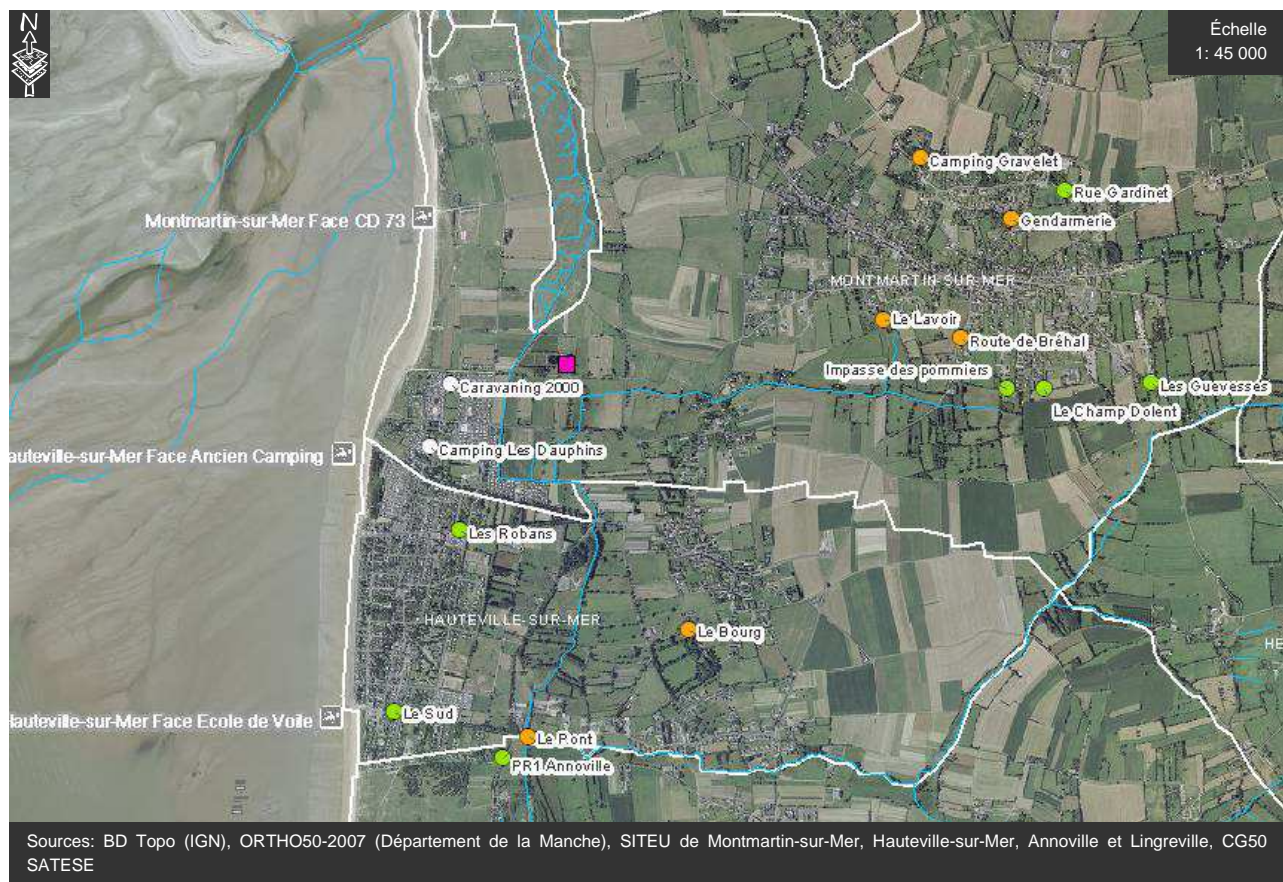
Figure 72 : Criticité globale des postes de refoulement sur le secteur de Montmartin-sur-Mer, Hauteville-sur-Mer et Annoville
