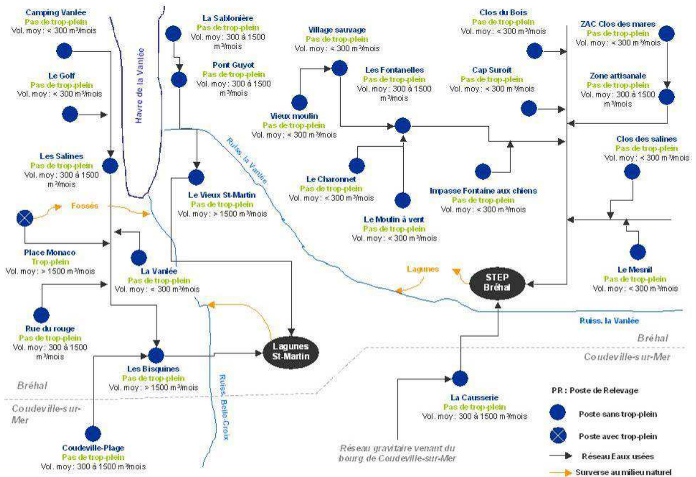
Figure 67 : Schéma conceptuel des réseaux d'assainissement sur le territoire de la commune de Bréhal
