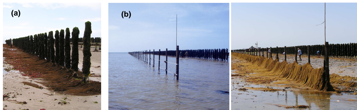
Figure 20 : (a) Amas de sargasses sur les pieux (mai 2005) – (b) vue sur le barrage pendant et après son installation Clichés transmis par le CRC NMN
