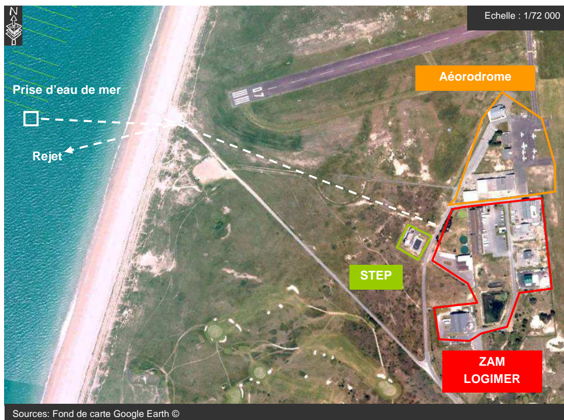
Figure 46 : Vue sur le rejet de la zone conchylicole de Bréville-sur-Mer
