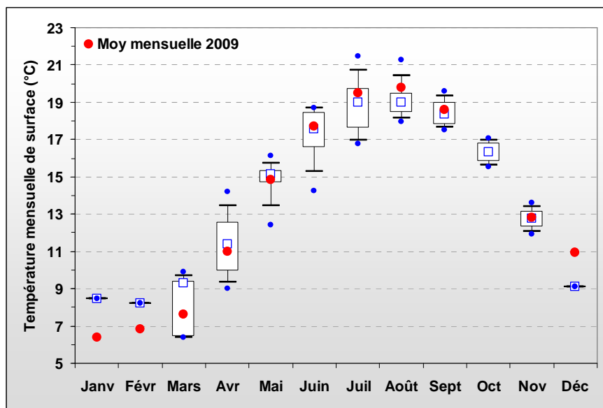
Figure 22: Distribution mensuelle de la température de l'eau sur le point suivi Coudeville 1 mille sur la période 2001-2009 (IFREMER-LERN)
