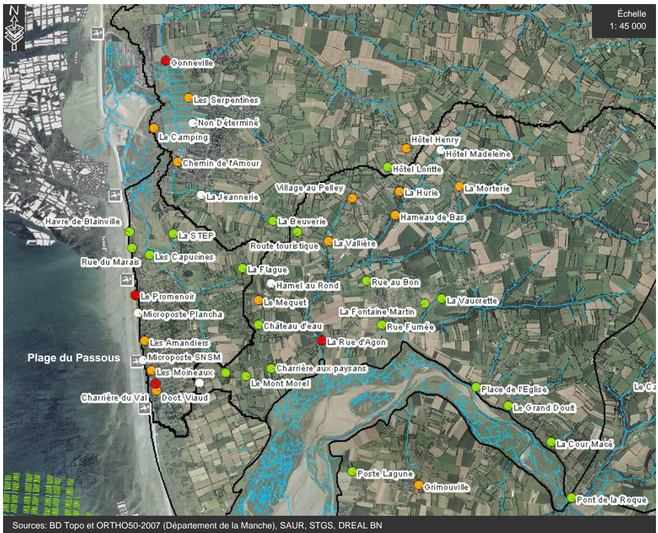
Figure 69 : Criticité globale des postes de refoulement sur le secteur de Blainville-sur-Mer / Agon-Coutainville / St-Malo-de-la-Lande / Tourville-sur-Sienne / Heugueville-sur-Sienne
