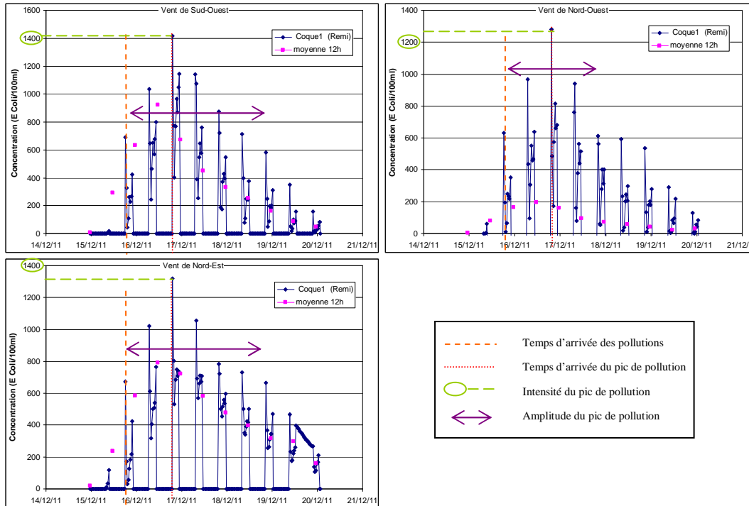
Figure 3-12 : Chroniques temporelles des concentrations dans l'eau de la zone classée 50-02 pour différentes conditions de vent et en temps de pluie semestrielle hivernal
