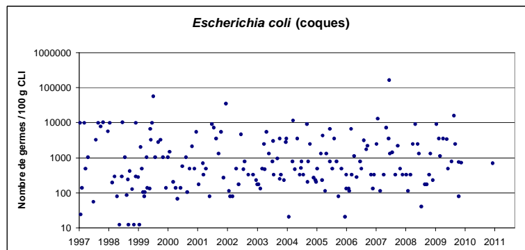
Figure 2-3 : Concentrations journalières en E.Coli des coques au point REMI du « Grand Vey »
